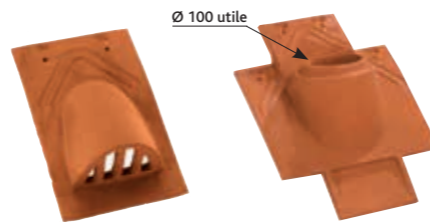
Tuile de ventilation 17 x 27 Phalempin (section de ventilation = 23 cm 2 ) Réf. 500.20 (1)
