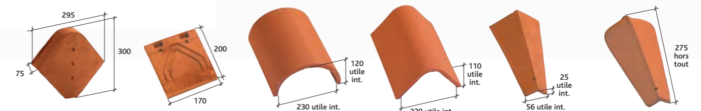
Fronton pour faîtière angulaire sans emboîtement Phalempin Réf. 808 (5)
