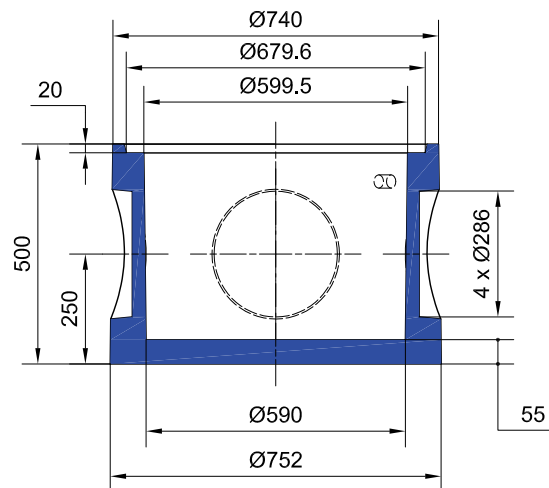
BOITE DE BRANCHEMENT CYLINDRIQUE TP Ø60 H : 50 Ep. 8 SANS COUVERCLE
