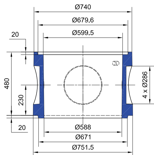
REHAUSSE H : 50 POUR BOITE DE BRANCHEMENT Ø60 CYLINDRIQUE
