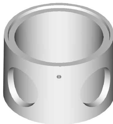
REHAUSSE H : 50 POUR BOITE DE BRANCHEMENT Ø60 CYLINDRIQUE
