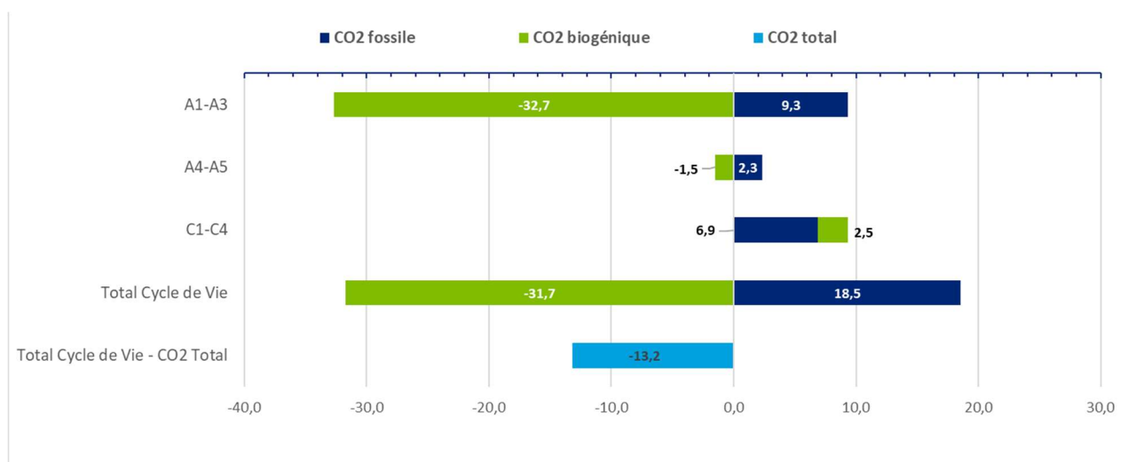
Figure 2 - Impacts en termes de changement climatique du panneau PARNATUR ISOLANT FIBRES DE BOIS 180 mm en considérant le carbone d'origine biogénique (kg eq. CO 2 ) – UF : 1m 2 d'isolation thermique pendant 50 ans
