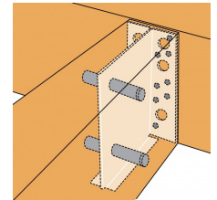
Assemblage solive sur poteau par broches
