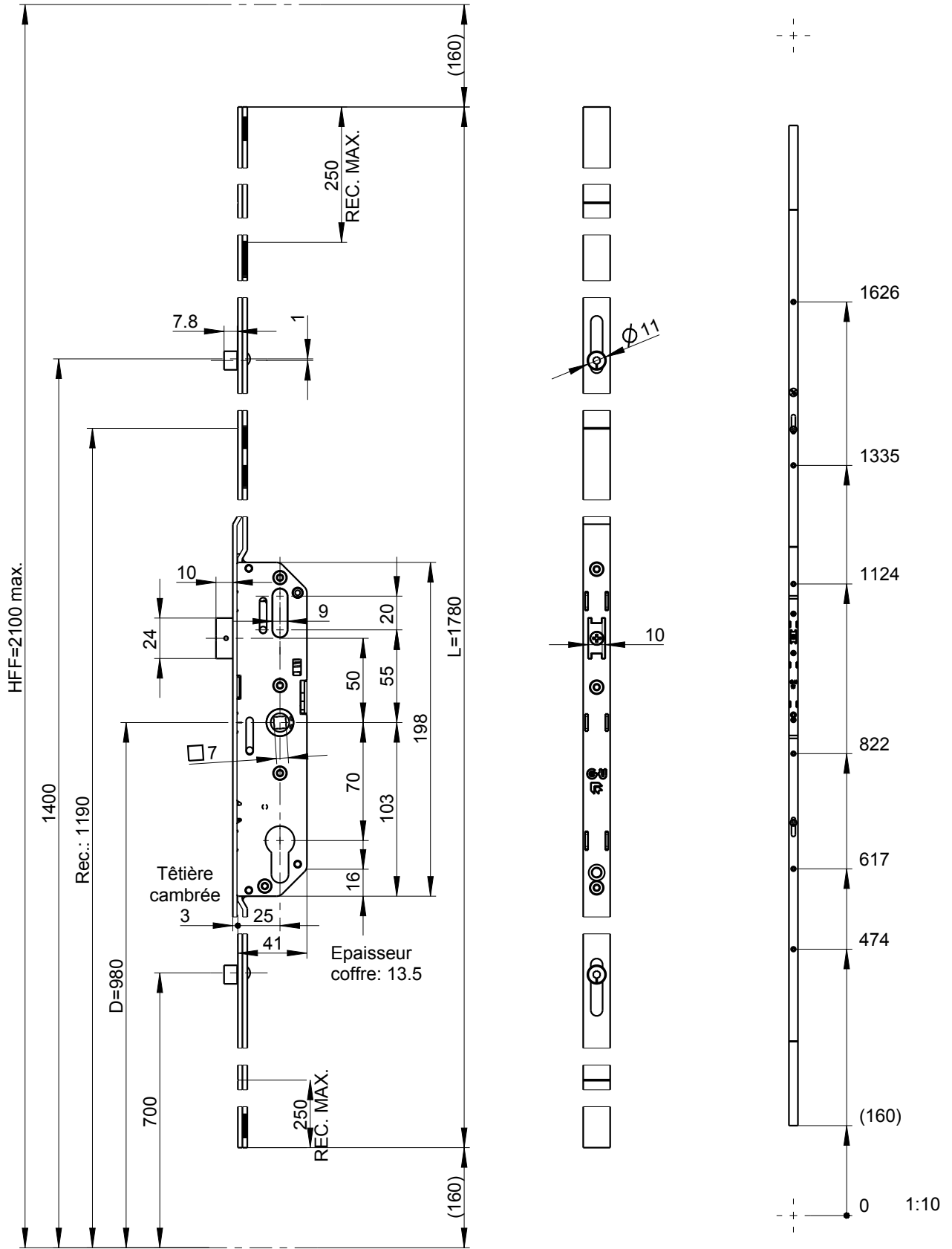
Crémone gauche représentée en position ouverture
