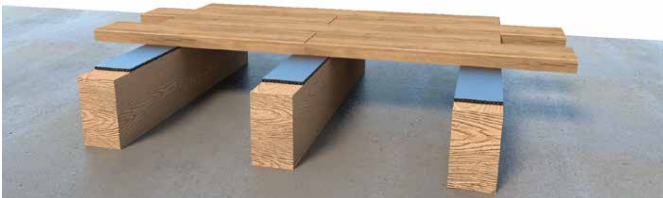
Pose du TRAMIBAND sur lambourde et plancher bois
