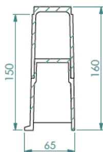
ULTIMA vue en coupe
