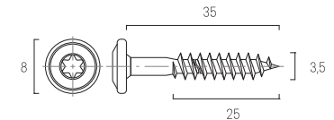
INOX-UP3.5X35-TX15-A2 Vis de fixation
