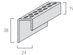
FS-261 Profil de finition U, perforé
