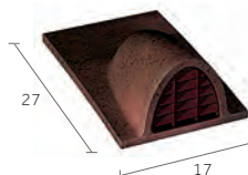
Tuile chatière avec grille (Ouverture 20 cm 2 )
