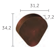
Fronton de rive à rabat pour faîtière demi-ronde
