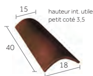
Arêtier d'about tige de botte de 33 (3 au ml)
