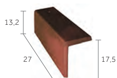
Demi-tuile de rive à rabat gauche (6 au ml)
