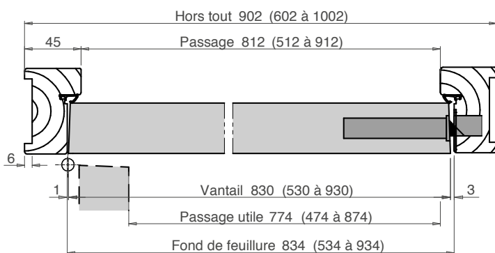
Ferrage représenté Paumelles 110x55 DU51
