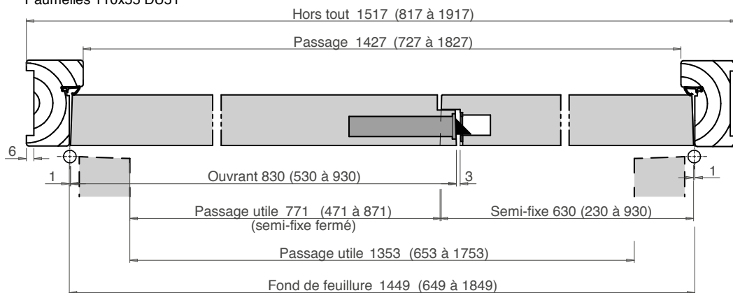
Ferrage représenté Paumelles 110x55 DU51
