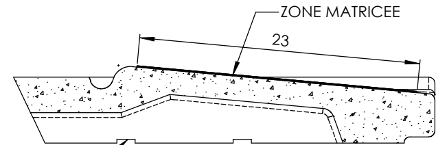
DÉTAIL B PROFIL DE LA RIGOLE
