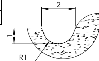
DÉTAIL B PROFIL DE LA RIGOLE
