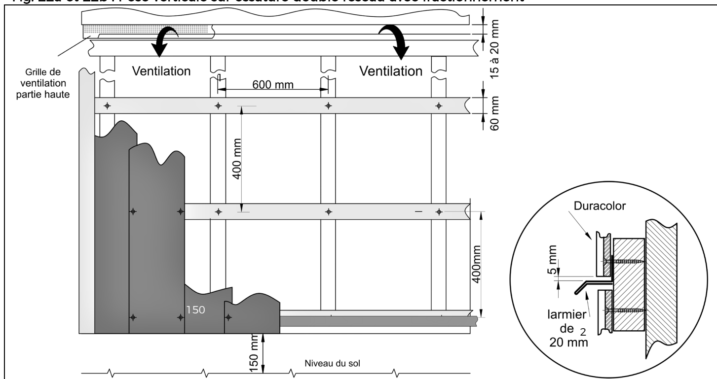
Fig. 22a et 22b : Pose verticale sur ossature double réseau avec fractionnement
