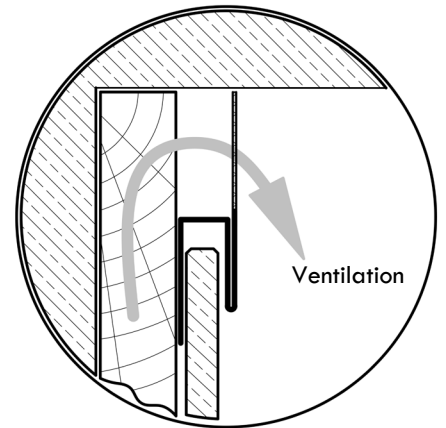
Fig. 18 - Ventilation en haut des façades : Grille de ventilation en partie haute : Grille perforée pour assurer la ventilation en haut des façades. A fixer derrière le dernier clin en partie haute Laisser la perforation de la ventilation apparente
