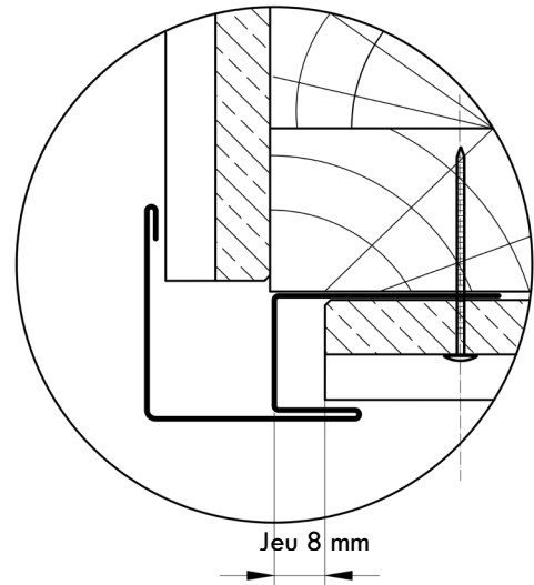
Fig. 18 - Ventilation en haut des façades : Grille de ventilation en partie haute : Grille perforée pour assurer la ventilation en haut des façades. A fixer derrière le dernier clin en partie haute Laisser la perforation de la ventilation apparente
