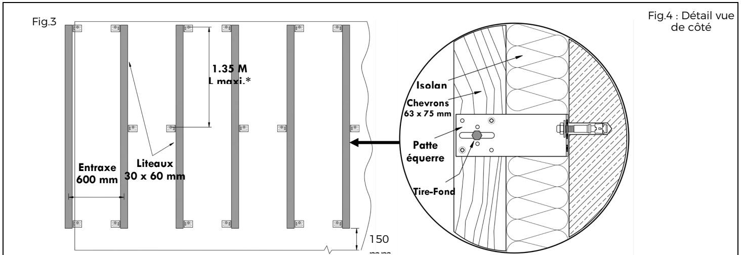
Fig. 4 et 5 : Ossature avec Isolation Thermique par l'extérieur
