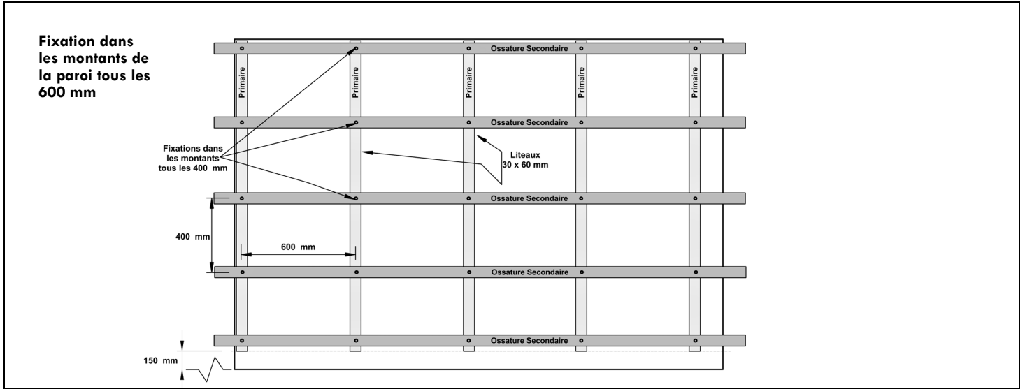
Fig.3 : Pose verticale du bardage - Ossature double réseau
