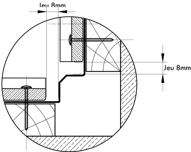
Fig. 14 - Angle rentrant : Profil coin intérieur continu
