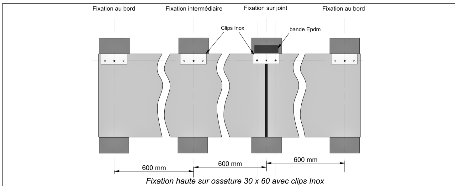
Fig.2 : Clips inox pose horizontale
