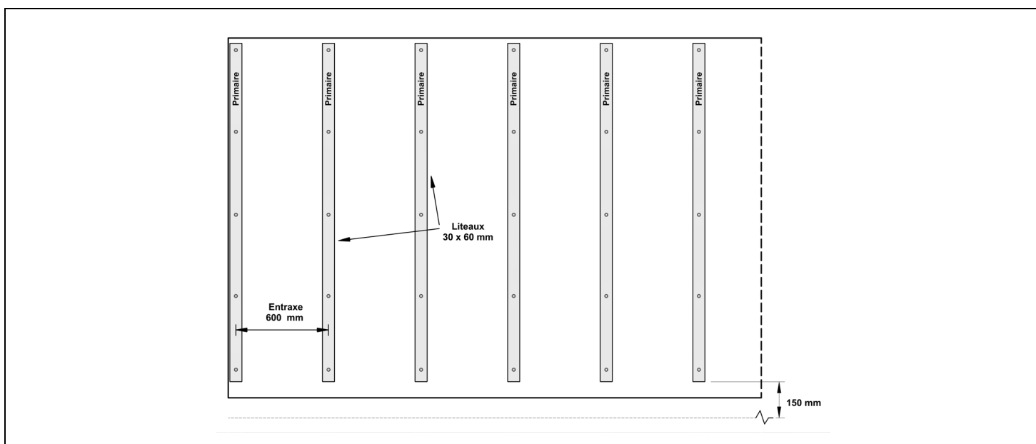
Fig.1: Pose horizontale du bardage sur maçonnerie et maison ossature bois - Ossature verticale simple réseau
