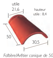
Faitière/Arêtier conique de 50
