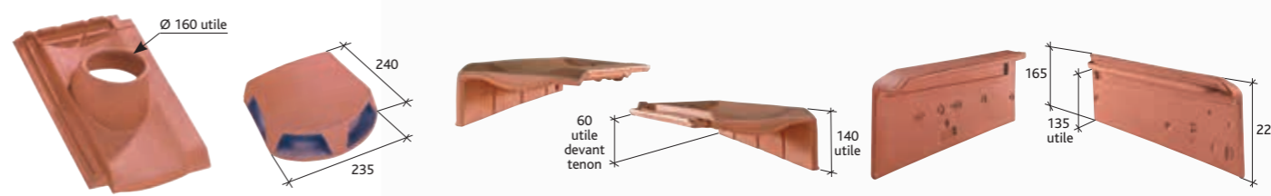
Tuile à douille H10 Ø 160 utile (conforme VMC) Réf. 203.32
