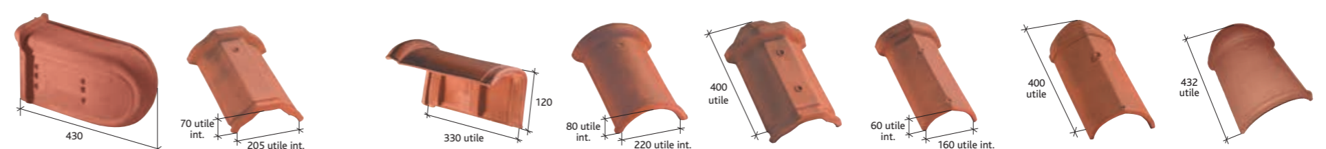
About de rive universelle gauche Réf. 1070 (3)
