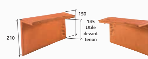
Rive individuelle gauche (4,6 par ml au pureau de 110 mm) Réf. 510.44
