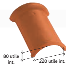
Faitière 1/2 ronde à emboîtement (2,5 au ml) Réf. 717 (2)
