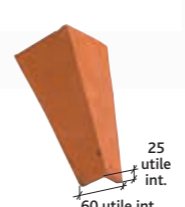
Arêtier angulaire sans emboîtement (9 à 10 au ml) Réf. 759
