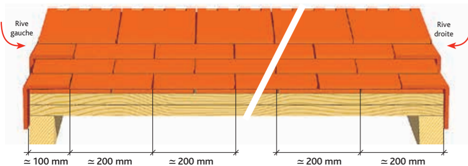
Faitière 1/2 ronde à emboîtement (2,5 au ml) Réf. 717 (2)
