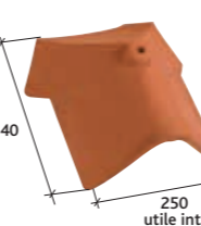
Rencontre porte poinçon 3 ouvertures, 1 faitière angulaire, 2 arêtiers angulaires Réf. 919 (8)
