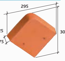
Fronton pour faitière angulaire sans emboîtement Réf. 808 (1)
