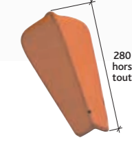
About d'arêtier angulaire sans emboîtement Réf. 864
