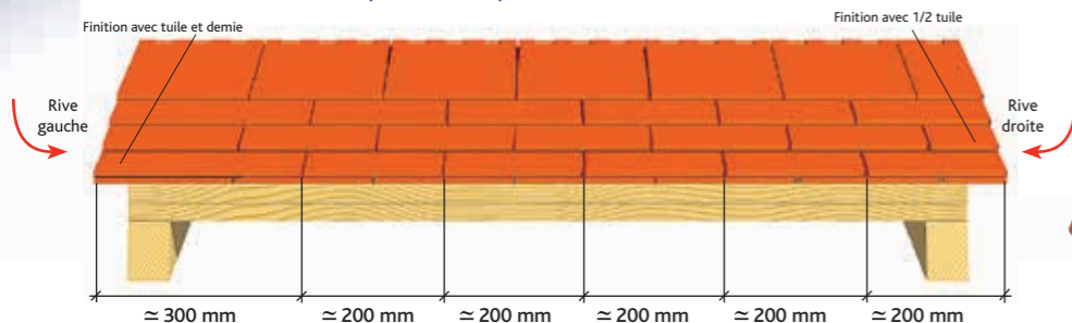
Tuile chatière Plate 20 x 30 kit 3 pièces Réf. 510.21
