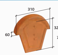
Fronton pour faitière 1/2 ronde à recouvrement Réf. 807
