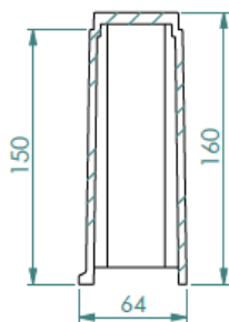
ULTIMA vue en coupe
